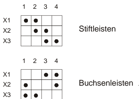
Abbildung 2: Klemmencodierung
